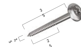
INOX-UP3.5X35-TX15-A2 Tornillo de montaje
