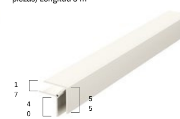
FS-261 Borde perforado Longitud 3 m
